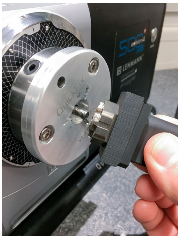
簡単なゼロ点クランプシステム（ここではSystem 3RのQuickFix）により、迅速なセットアップを実現します。
