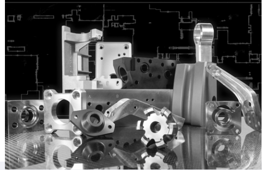
Breit aufgestellt: HS Fertigungstechnik liefert Bauteile von klein bis groß aus unterschiedlichsten Werkstoffen. (Bild: HS)
