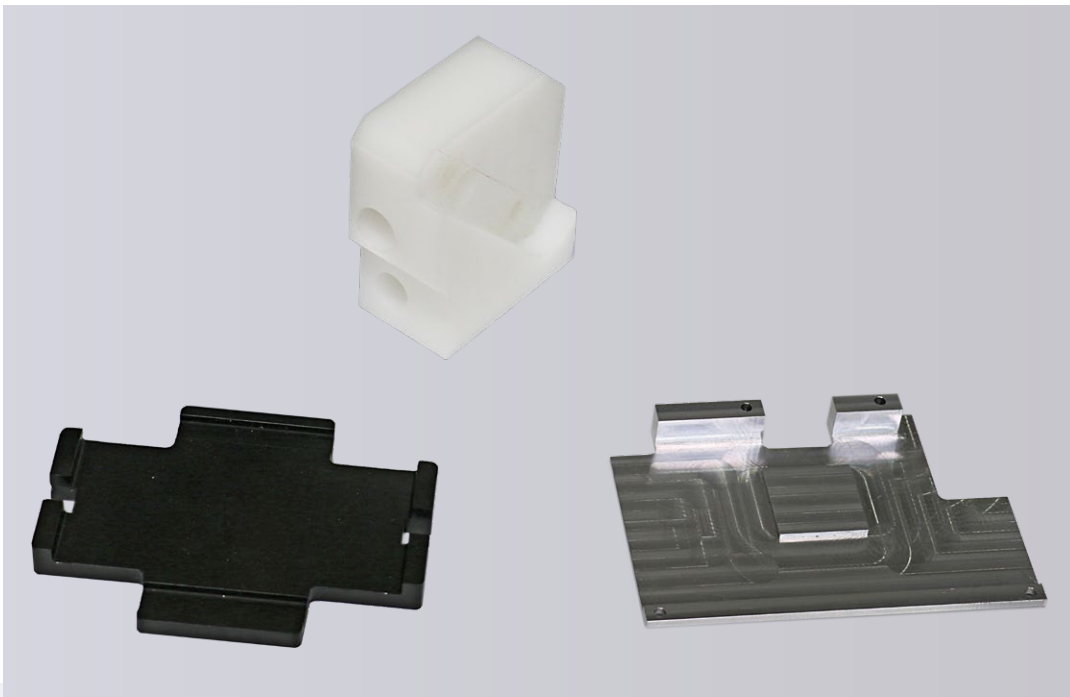
HS Fertigungstechnik nutzt die Fanuc Robodrill mit zweiachsigen pL Drehtisch zu 98 Prozent für Kleinteile bis 100 mm aus Aluminium und Kunststoff.
